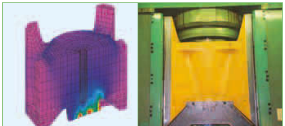
Kaltfließpresse (25 MN): Neuer FEM optimierter Stößel und fertig eingebauter neuer Stößel
